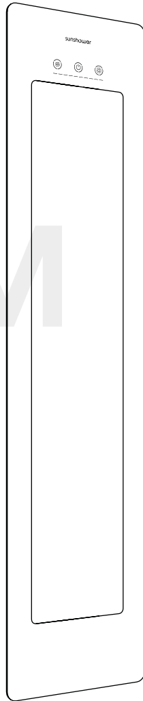
Sunshower ONE /M - IR Sunshower PLUS /M - IR+UV Sklo – dl. 1400 x š. 330 mm Rozmery zabudovaného zariadenia – dl. 1319 x š. 263 mm vstavaný / nástenný / rohový
